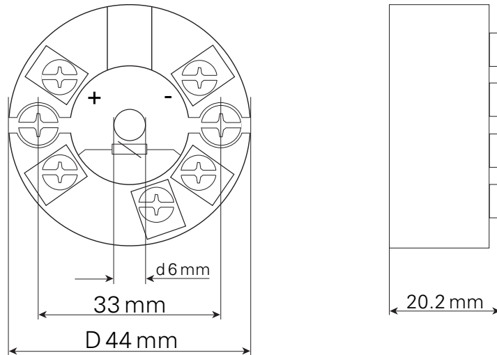
Figure 2-7 Dimensions mécaniques
