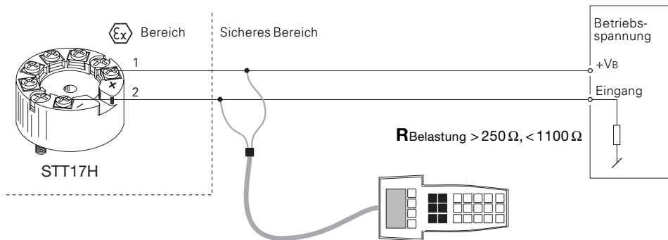
Figure 3-5 HART® Datenaustauschgerät
