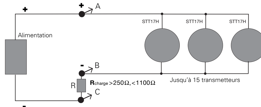
Figure 2-6 Raccordement des transmetteurs en multi-adressage
